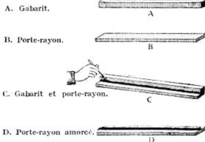
Gabarit pour amorcer les porte-rayons.
